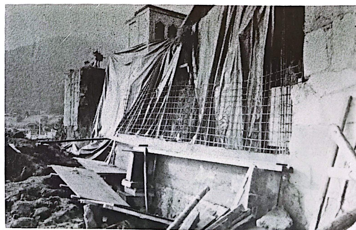
Trabajos de la barda perimetral, muros y gavetas del panteón de Mazatlán.
